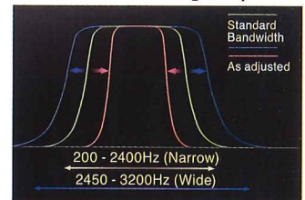
IF WIDTH function (LSB/USB)
