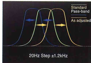
IF SHIFT function
